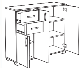
Roma 3 112,5x37x95cm ID 1403**
